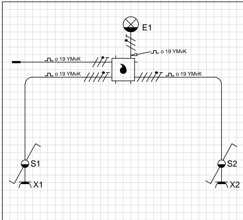
Installatieschema
