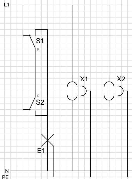
Stroomkringschema
